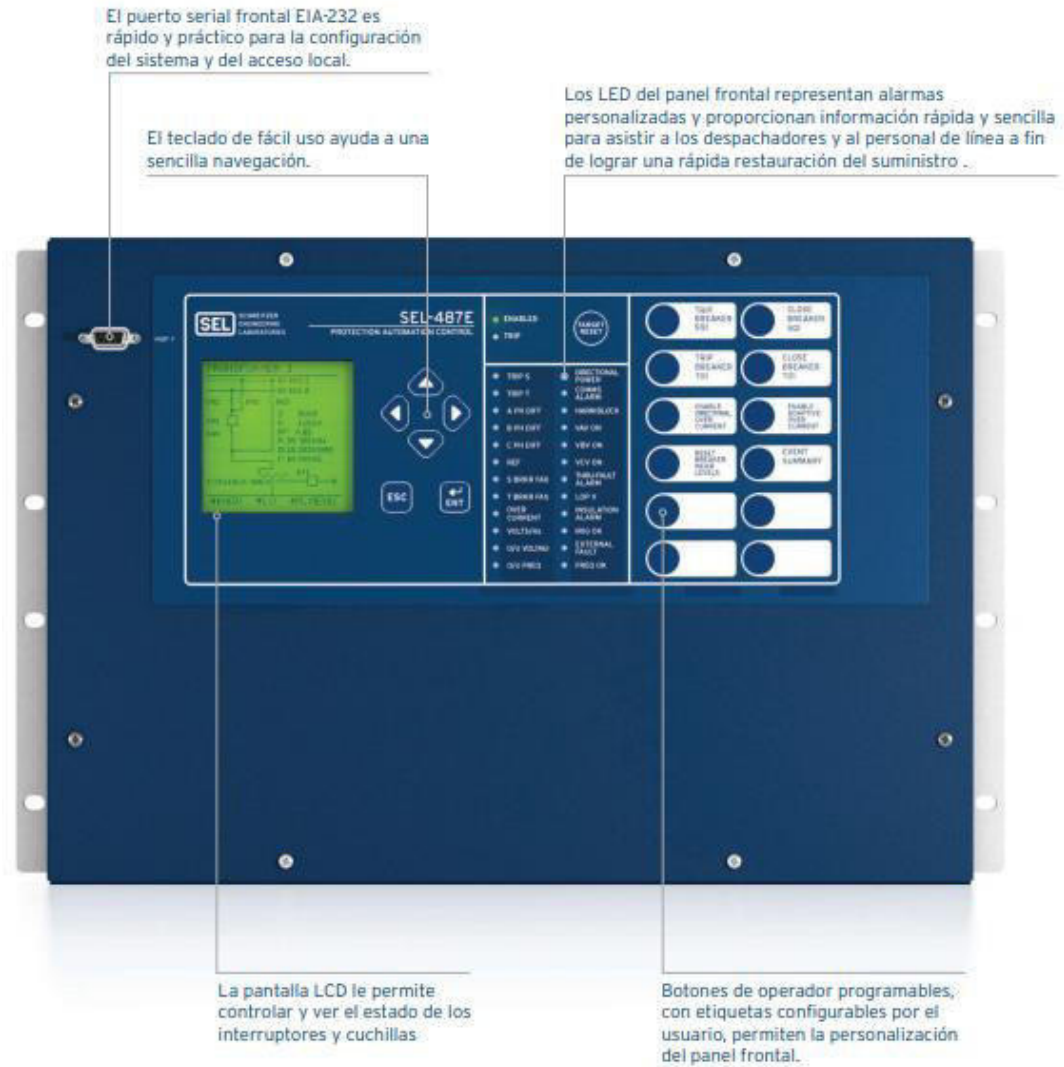
Figura 61 - Vista Frontal, Relé SEL-487E
