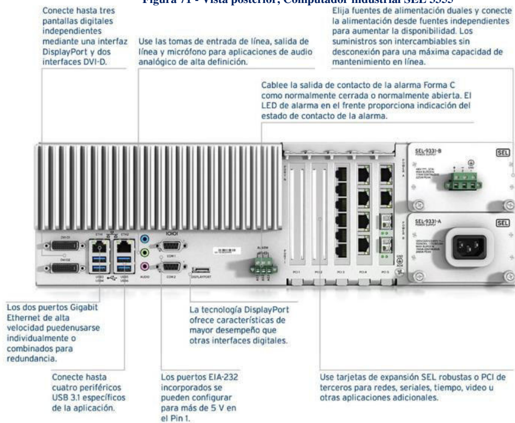
Figura 71 - Vista posterior, Computador industrial SEL 3355
