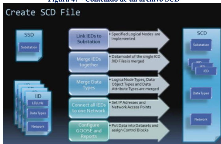
Figura 47 - Contenido de un archivo SCD
