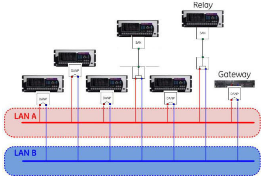
Figura 36 - Esquema simple aplicando PRP
