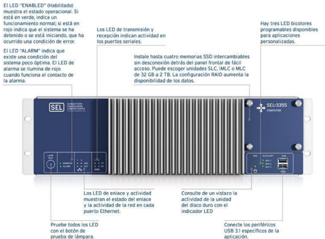
Figura 70 - Vista frontal, Computador industrial SEL 3355
