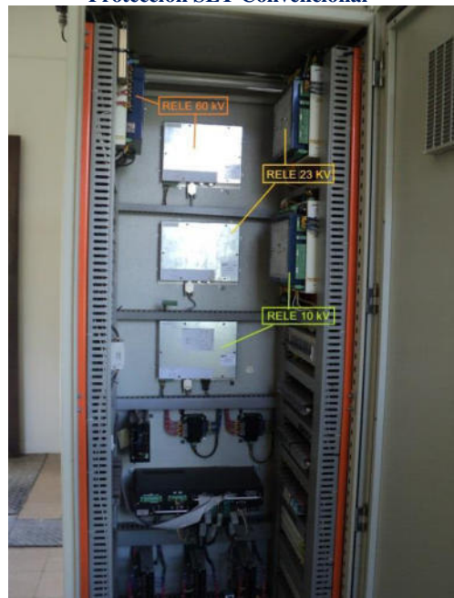
Figura 51 - Vista interior, Tablero Control y Protección SET Convencional
