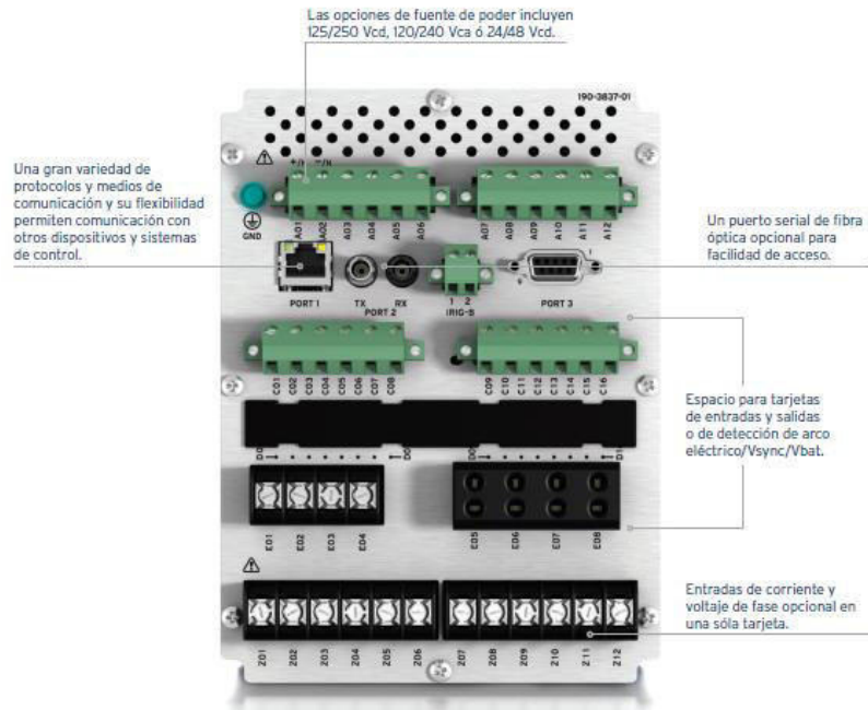
Figura 59 - Vista posterior, Relé de protección SEL-751
