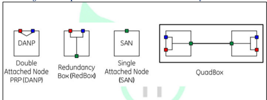
Figura 38 - Dispositivos usados en redes redundantes PRP y HSR
