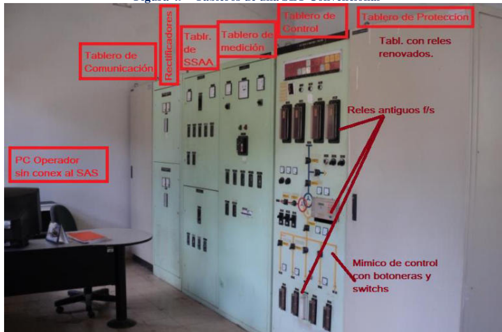
Figura 49 - Tableros de una SET Convencional
