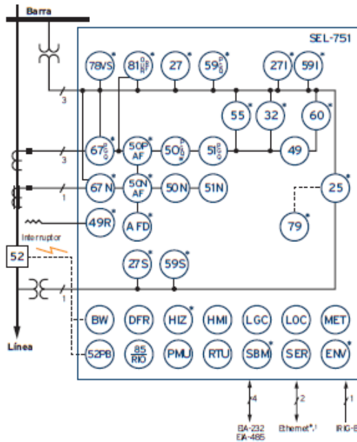
Figura 60 - Funciones de protección de relé SEL-751
