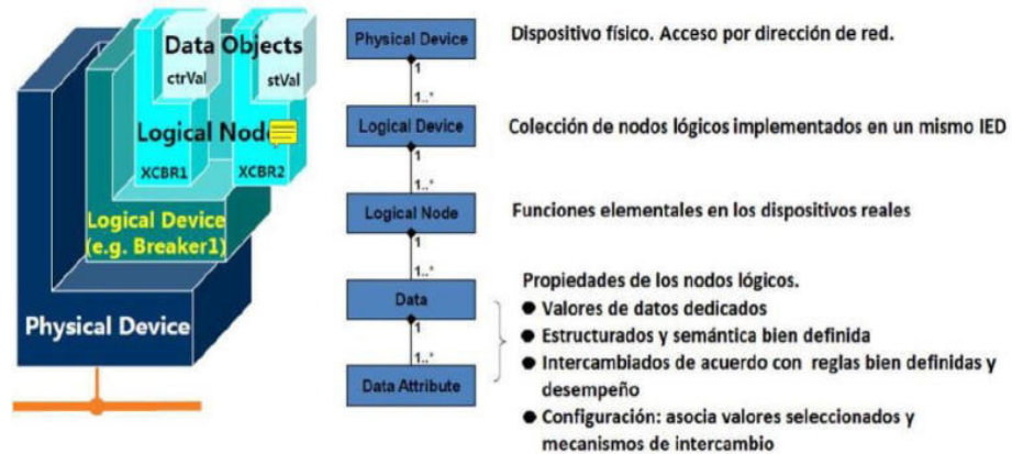
Figura 14 - Descomposición funcional y jerárquica de un dispositivo
