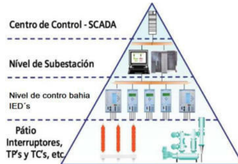
Figura 8 Niveles jerárquicos de control en una SET
