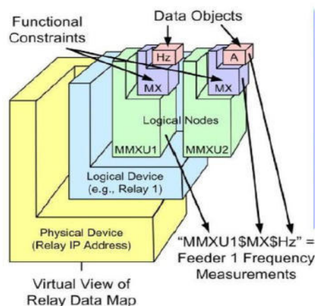
Figura 9 - Modelo de datos del estándar IEC 61850
