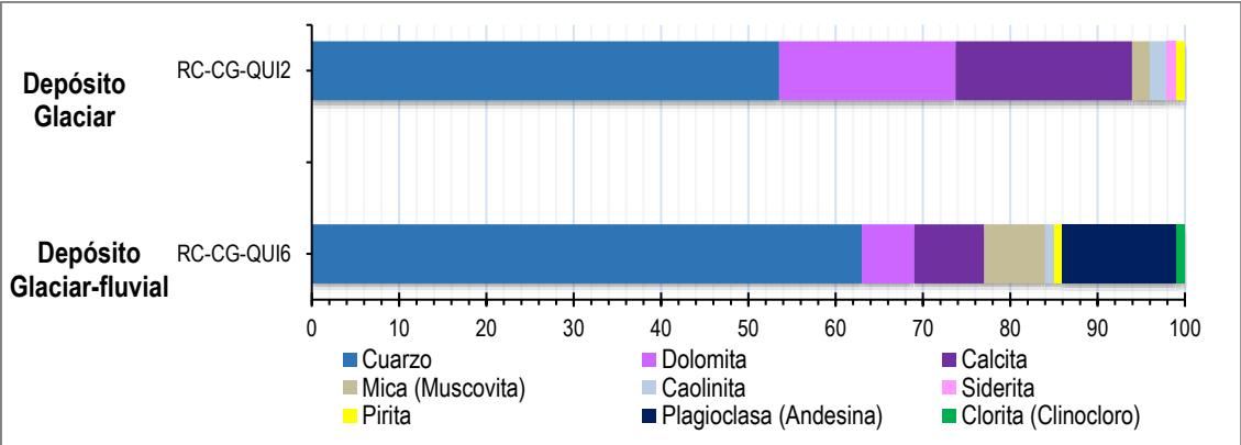
Figura 5.36. Composición mineralógica por DRX de los depósitos glaciar y glaciar-fluvial aledaño al CP Quiulacocha
