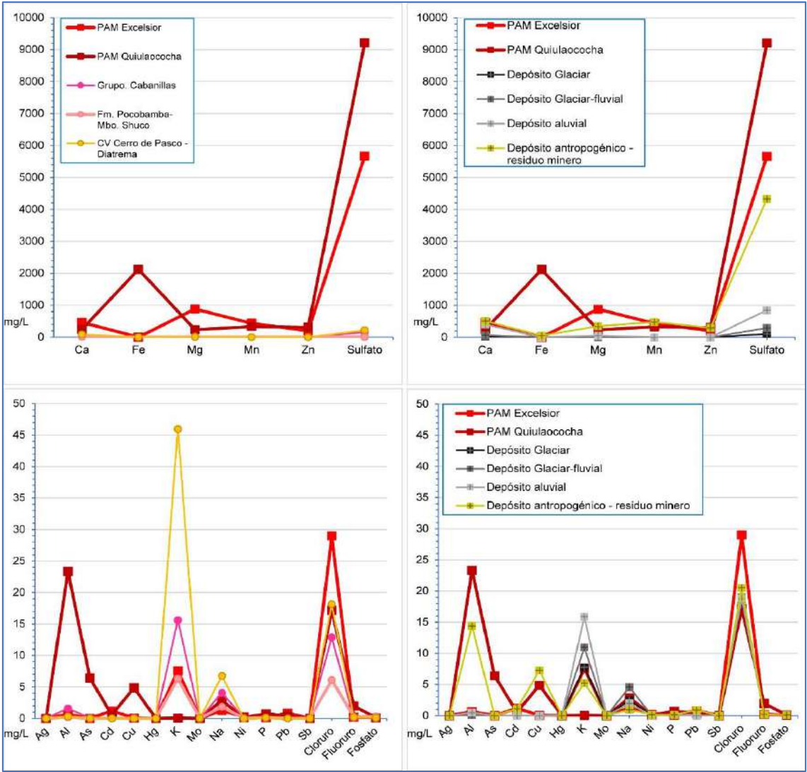
Figura 6.7. Comparación del potencial para lixiviar iones de las unidades litológicas, comparados con el material de los PAM Excelsior y Quiulacocha
