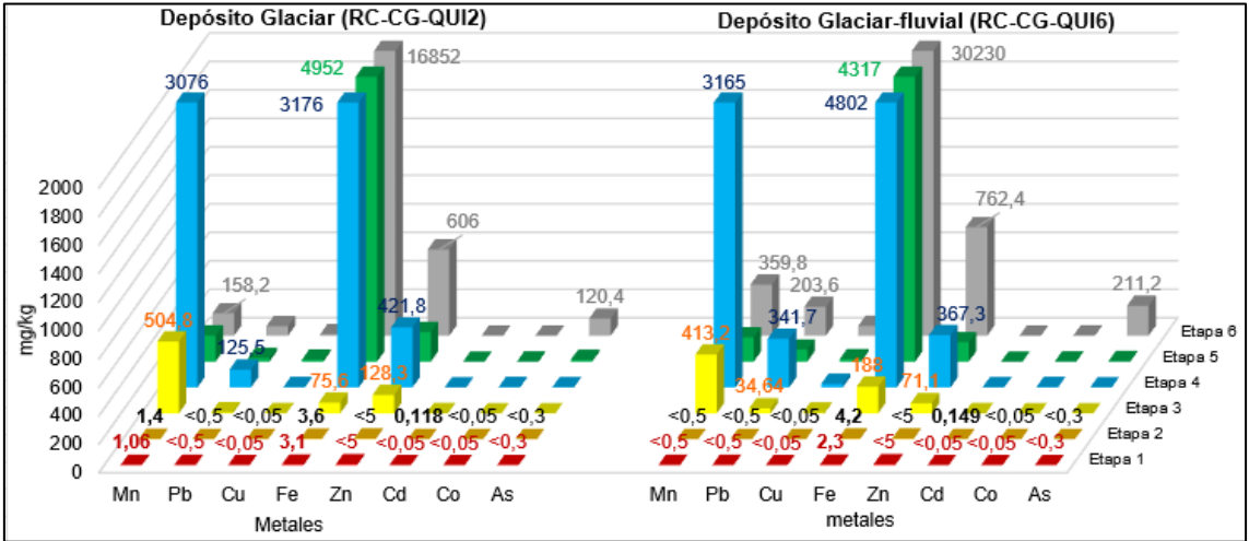
Figura 5.29. Concentración de metales de las extracciones secuenciales por la prueba de Tessier de los depósitos cuaternarios aledaños al PAM Quiulacocha
