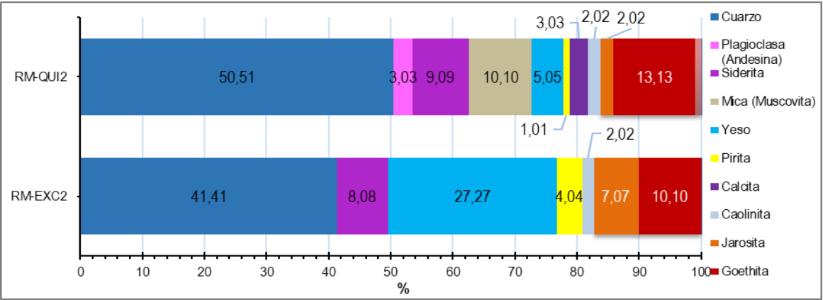
Figura 5.37. Composición mineralógica por DRX de los depósitos antropogénicos-residuos mineros aledaños a los CP Champamarca y Quiulacocha.
