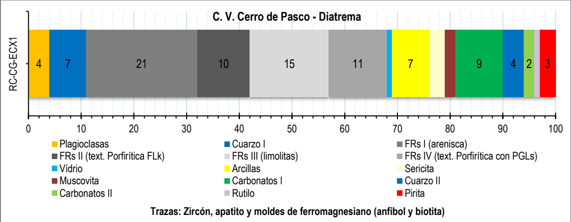
Figura 5.33. Composición mineralógica por petromineragrafía del diatrema del CV Cerro de Pasco aledaño al PAM Excelsior
