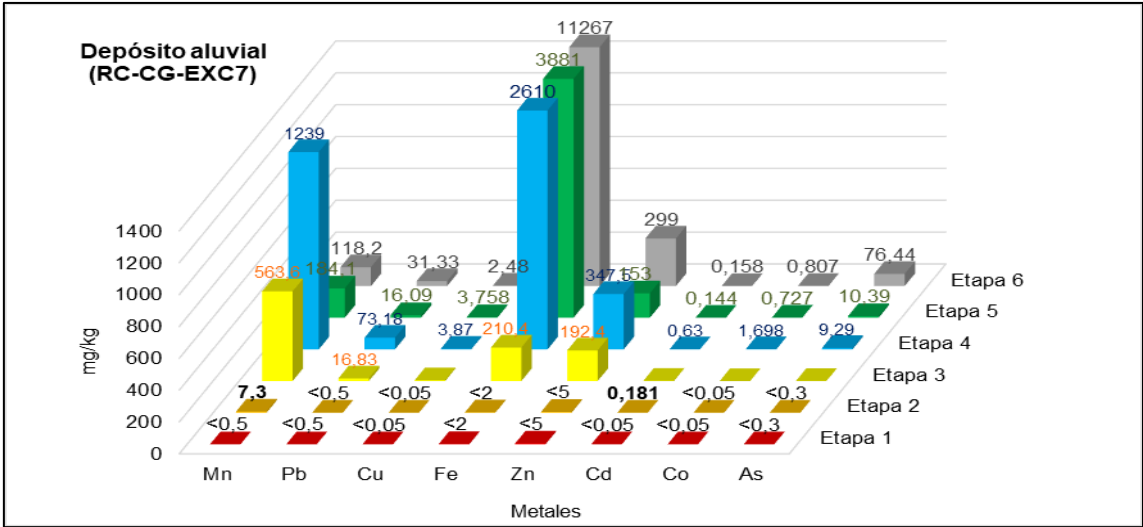
Figura 5.28. Concentración de metales de las extracciones secuenciales por la prueba de Tessier del depósito aluvial aledaño al CP Champamarca
