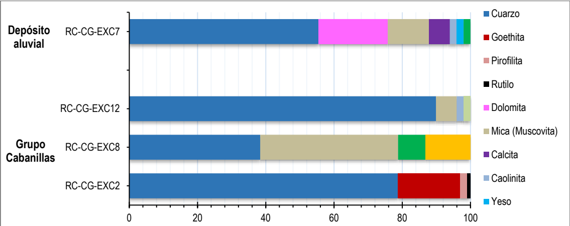
Figura 5.31. Composición mineralógica por DRX del Grupo Cabanillas y depósito aluvial aledaños al PAM Excelsior
