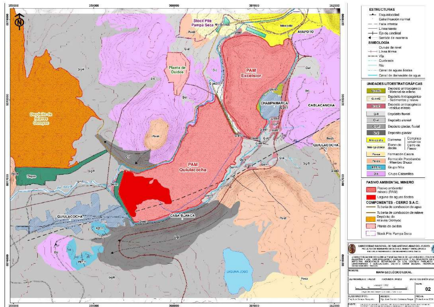
Figura 5.2. Mapa geológico local del área de estudio
