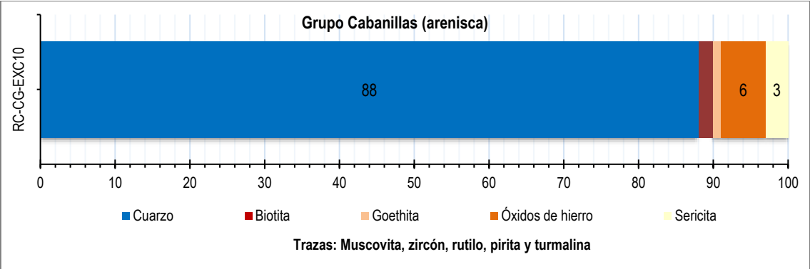
Figura 5.32. Composición mineralógica por petromineragrafía del Grupo Cabanillas aledaño al PAM Excelsior
